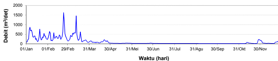
HIDROGRAF DEBIT HARIAN (m 3 /dt) S.BENGAWAN SOLO-BALUN TAHUN 2018
