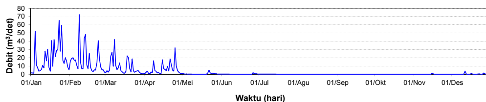
HIDROGRAF DEBIT HARIAN (m 3 /dt) S.DENGKENG-JARUM TAHUN 2018
