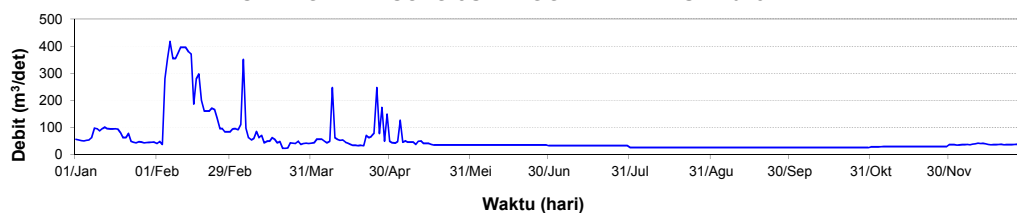
HIDROGRAF DEBIT HARIAN (m 3 /dt) S.BENGAWAN SOLO-JURANGGEMPAL TAHUN 2018
