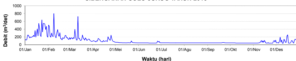
HIDROGRAF DEBIT HARIAN (m 3 /dt) S.BENGAWAN SOLO-JURUG TAHUN 2018
