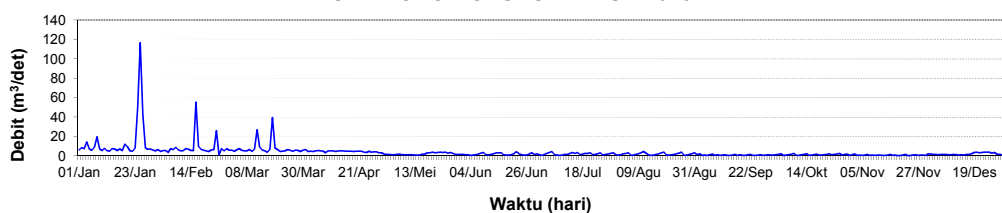
HIDROGRAF DEBIT HARIAN (m 3 /dt) S.CEMORO-NGRUKUN TAHUN 2018
