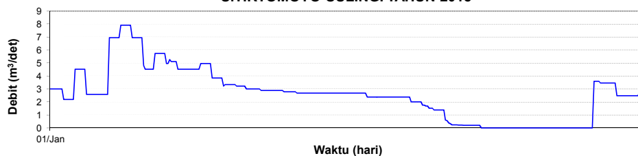
HIDROGRAF DEBIT HARIAN (m 3 /dt) S.TIRTOMOYO-SULINGI TAHUN 2018
